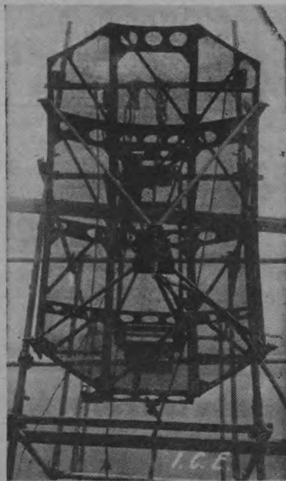
ANTENA PARABOLICA DIRECCIONAL. Mediante esta antena son captadas las señales de frecuencia ultra alta, mediante las cuales se establecerá la red de telecomunicaciones en todo el país con centrales completamente automáticas. Esto es parte del programa de telecomunicaciones, puesto en marcha por el ICE.
